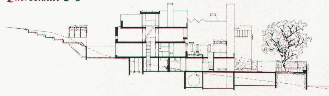
Querschnitt 2-2
