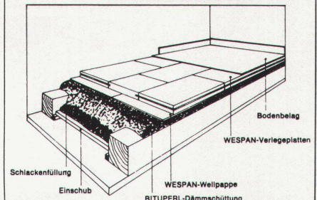
auf Holzbalkendecken
