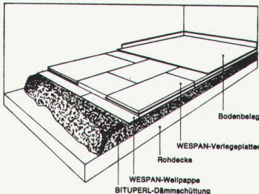
auf Rohdecken
