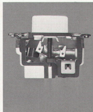
Gekapselter Sockel staubgeschützt und berührungssicher
