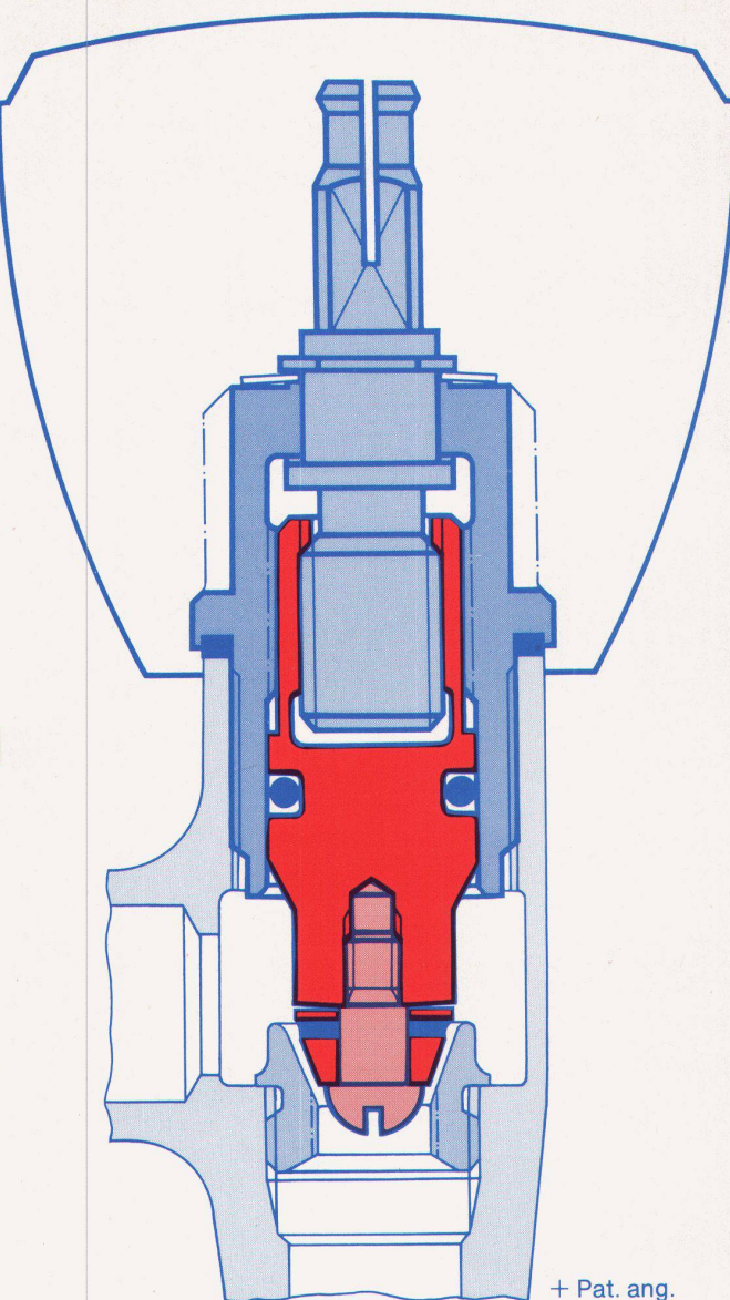
Stellung « offen »
