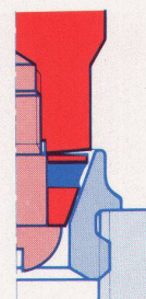
beim Schliessen Regulierkonus aufgesetzt, Dichtung nicht gepresst
