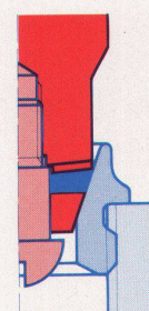
Stellung «geschlossen» Regulierkonus aufgesetzt, Dichtung achsial gepresst, metallischer Anschlag
