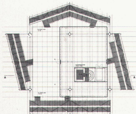
Grundriss 3. Betriebsgeschoss
