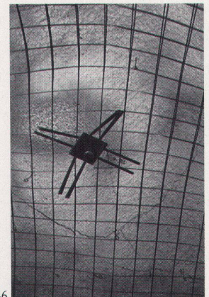
46 VSL-Anker, 2 m tief, je 10 m 2 Felsdecke
