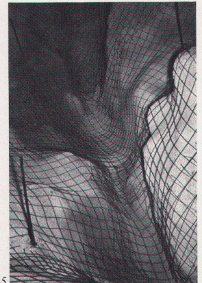
45 Netzarmerung auf erster Gunitsschicht
