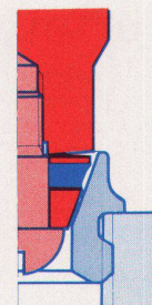
beim Schliessen Regulierkonus aufgesetzt, Dichtung nicht gepresst
