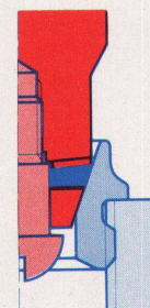
Stellung «geschlossen» Regulierkonus aufgesetzt, Dichtung achsial gepresst, metallischer Anschlag
