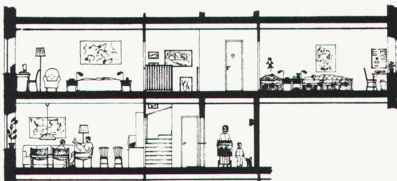
Schnitt durch eine zweigeschossige Fünzimmerwohnung
