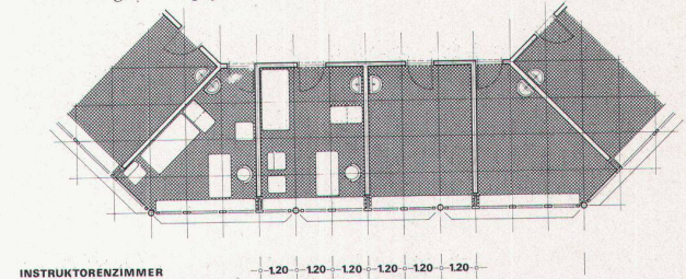
Möblierungen «Triptyk» 1:250
