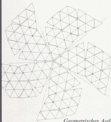
Geometrischer Aufbau der Kuppel
