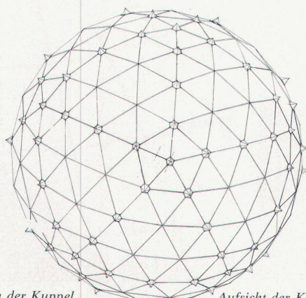
Geometrischer Aufbau der Kuppel
