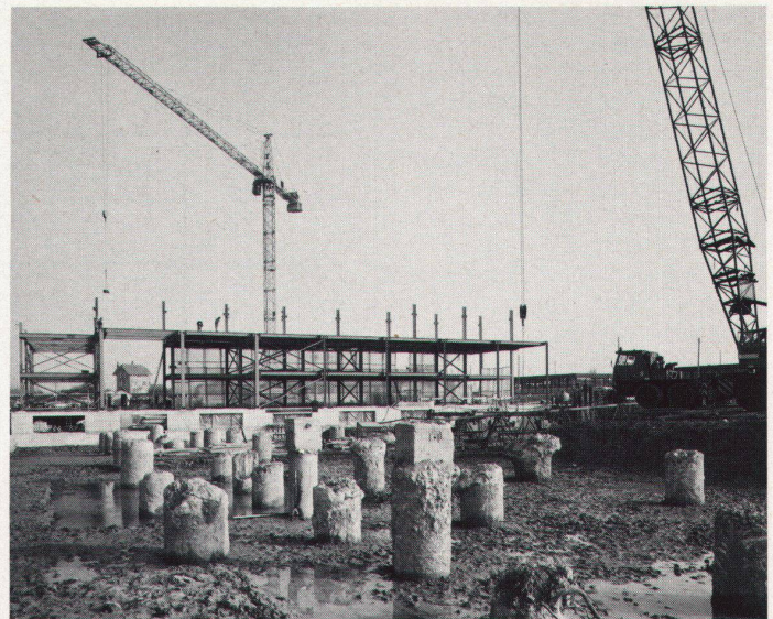
Construction de la galerie d'alimentation primaire
