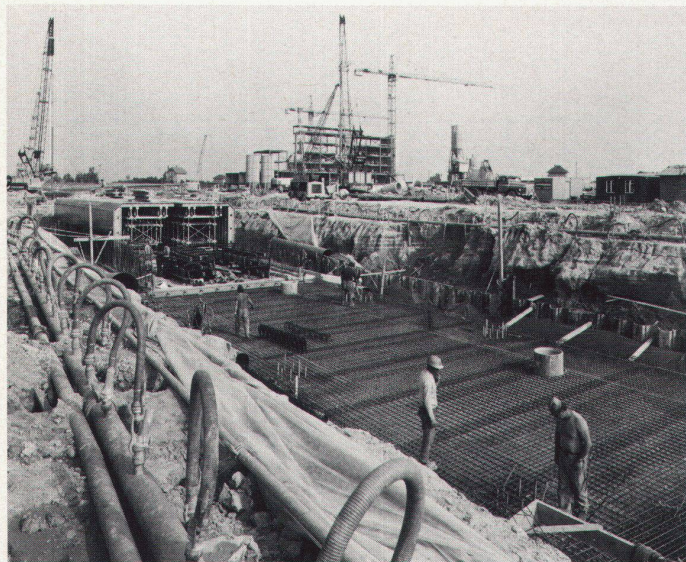
Pieux et charpente métallique
