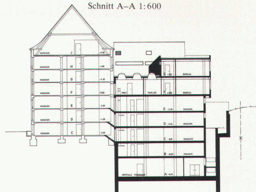
Schnitt A-A 1:600
