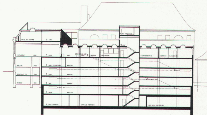
Schnitt B–B 1:600
