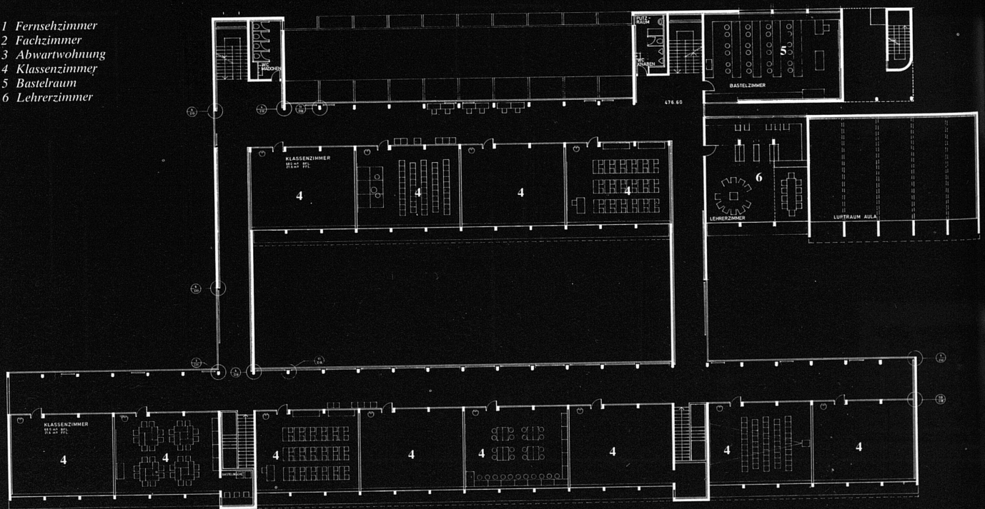
Grundriss 1. Obergeschoss
