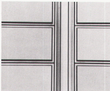
Grundriss und Schnitt Fassadenelement/Element de façade en plan et coupe/Plan and section of exterior panel
