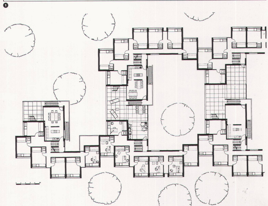
1 Studentenzimmer, Grundriss und Ansichten der Wohneinheit / Chambre d'étudiant, plan et élévations de l'unité habitable / Student's room, plan and elevation views of the residence unit
