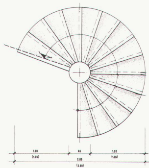
Grundriss Typ «Winkel»
