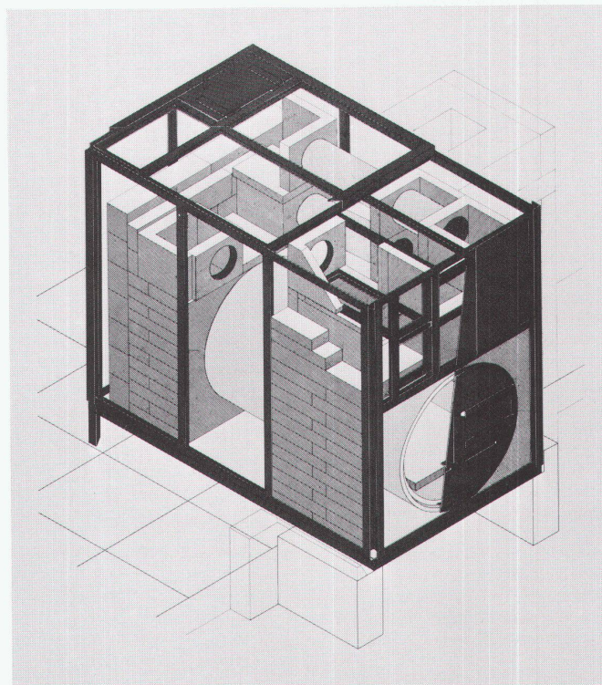
6-9 Der neue Speicherofen in seinem Aufbau und Aussehen
