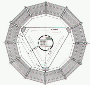
7 Grundriss (Typ FMT 216)
