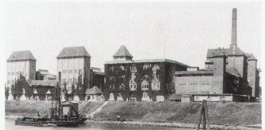
Kaffee-fabrik in Eisenbeton, Hugo Wagner, Bremen 1907
