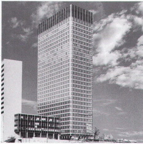
Tour Nobel Paris 1967/69, Vor-Hängefassade Jean Prouvé C.I.M.T.
