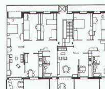
Neue Wohnüberbauungen 3: Luzernerring, Basel, 1993; Architekten: Michael Alder und Partner. Struktur und Typengrundriss. Anpassbare Grundrisse mit wählbaren Trennwänden, unter- schiedliche Grundrisse, grosse Küche mit Essplatz, veränderbare Raumbeziehung mit Schiebewand, grosses Bad mit separatem WC, drei verschieden nutzbare Balkone, abge- schlossener interner Eingangsbereich
