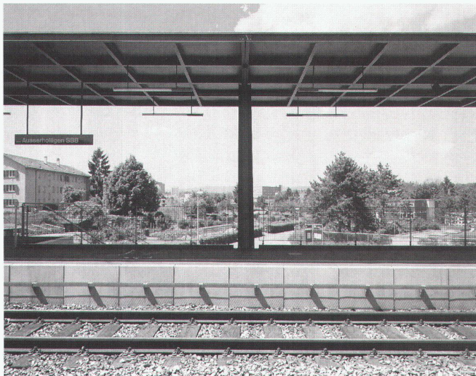
Berner S-Bahn-Station Ausserholigen, Architekt: Rolf Mühlethaler, Bern
