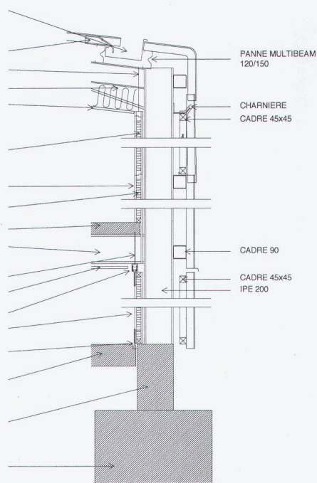
Details Innenwand zum Wintergarten und Aussenwand Strassenseite ▷ Détails paroi intérieure vers le jardin d'hiver et paroi extérieure côté rue ▷ Details of the interior wall to the winter garden, and the street side exterior wall
