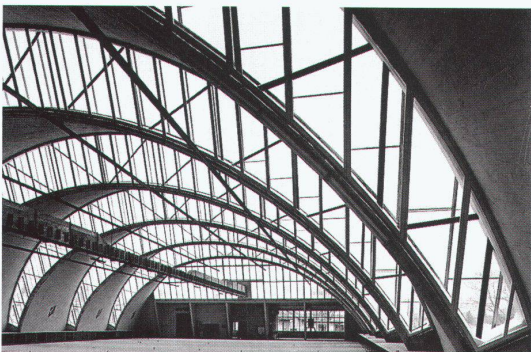
Ennenda, Hänggigturm: Heinz Hossdorf, Fabrikhalle Gummibandweberei Gossau, 1954/55 (Architekten Danzeisen und Voser, St. Gallen)
