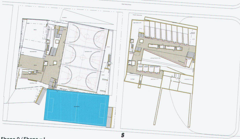
Ebene 0/ Ebene - 1
