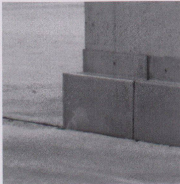
Detail Dachanschluss (Fotos: Ruedi Walti)
