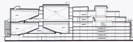
Längsschnitt
