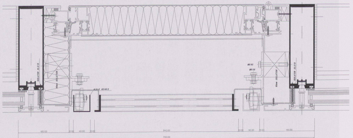
Fassade: Horizontal-Schnitt, 1:5
