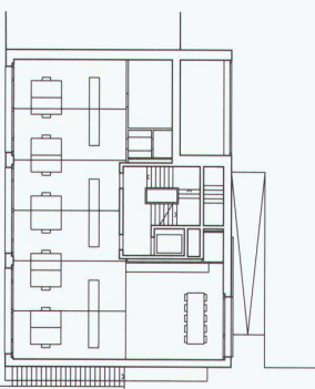
1. Obergeschoss
