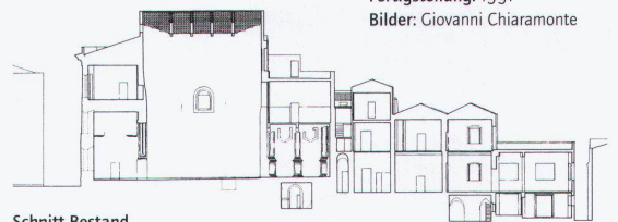
Schnitt Bestand
