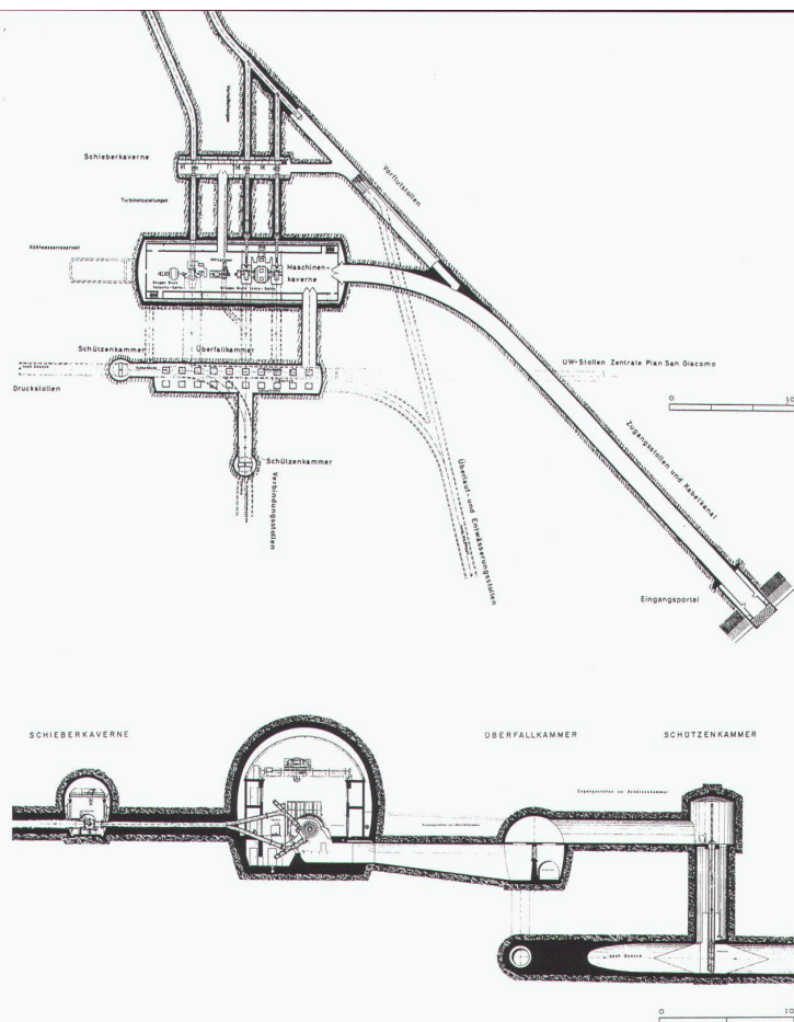
Übersichtsplan und Querschnitt der Zentrale Spina. – Bild aus: Conradin Clavuot, Jürg Ragetti, Die Kraftwerksbauten im Kanton Graubünden, Chur
