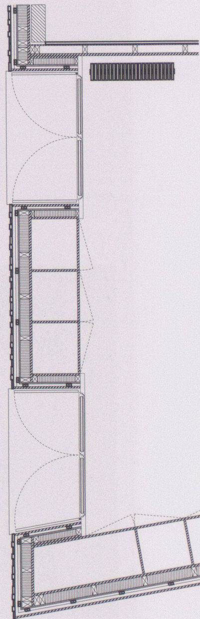
Horizontalschnitt
