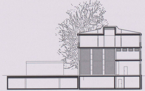
Querschnitt
