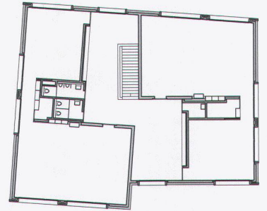
Obergeschoss
