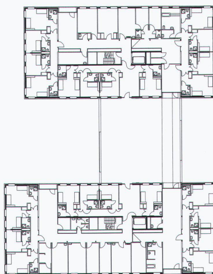
Grundriss 2. OG
