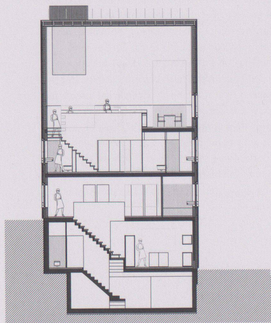
coupe
