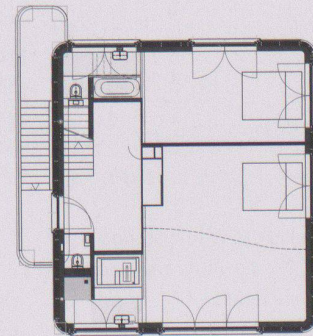
niveau 2
