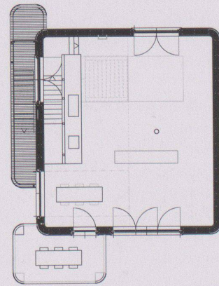
niveau 3
