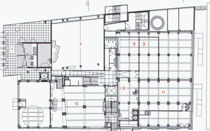
Erdgeschoss
