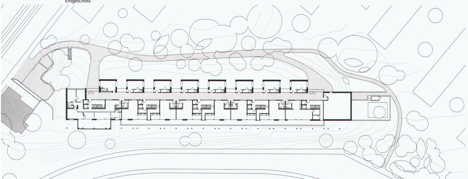
Erdegesschoss
