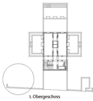
1. Obergeschoss
