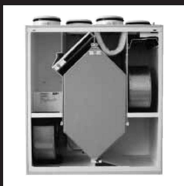
KWL-Lüftungssystem
