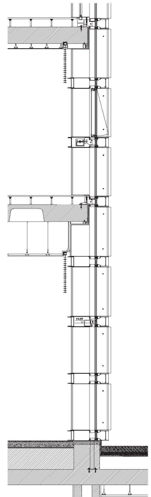
Detailschnitt Turm
