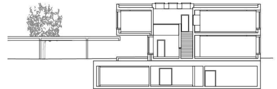
Schnitt 3
