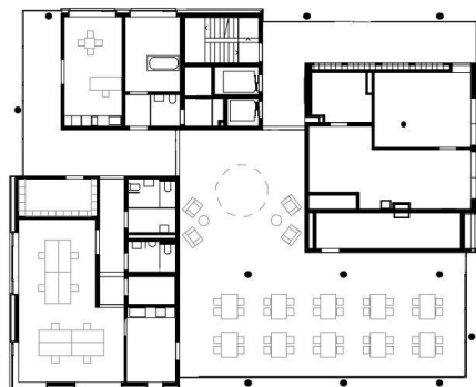
Erdgeschoss
