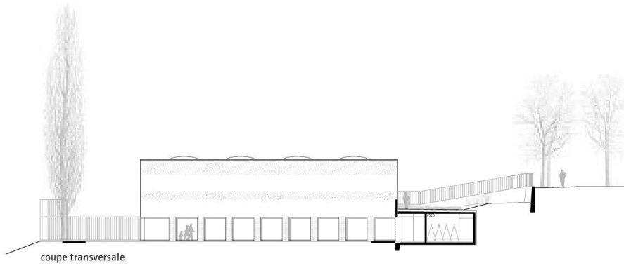
coupe transversale
