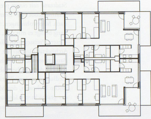
2. Obergeschoss
