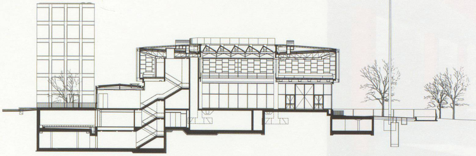
Schnitt A
