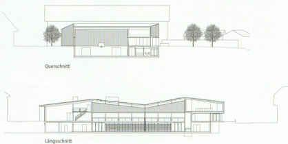
Längsschnitt
