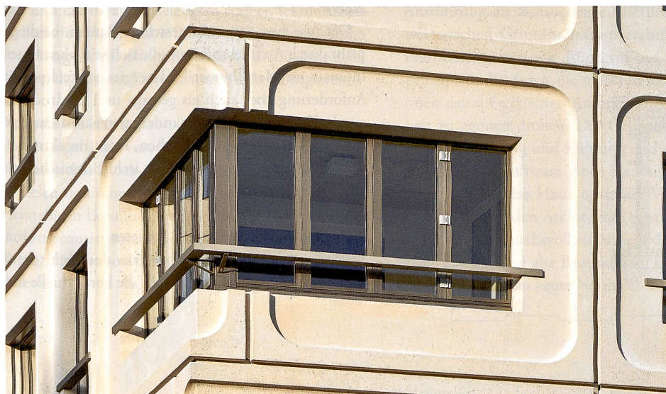
Die vorfabrizierten tragenden Betonelemente wurden geschossweise versetzt und mit den Deckenstirnen kraftschlüssig ausbetoniert. Die Sandwichelemente wirken als Rahmen. Sowohl Stoss- wie Lagerfugen sind überlappend ausgebildet, so dass auf sichtbare Silikonbänder verzichtet werden kann. Die Fuge erhält als grosszügiges Schattenband eine gestalterische Wichtigkeit in der gesamten tektonischen Formulierung und unterstützt bis in die Nahbetrachtung die starke Plastizität im Ausdruck des Gebäudes. – Bild: Jürg Zimmermann
