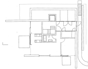
Erdgeschoss «Gartenvilla»
