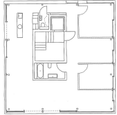
3. Obergeschoss «Pavillon»
