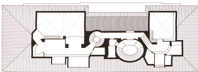
Galeriegesschoss im Dach
